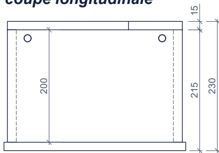
kelder met afdekplaat cave avec couvercle
