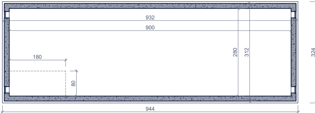
bovenaanzicht vue de dessus
